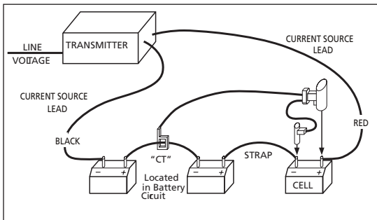
Figura 2. Configuración común de prueba
