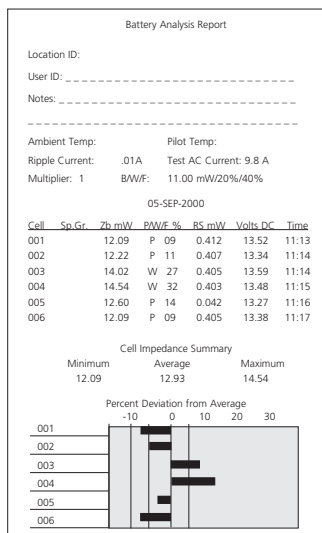
Figura 1. Modelo de informe de análisis de baterías
