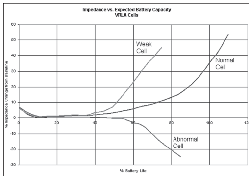
Figura 4. La impedancia aumenta con la edad (y debilitamiento) de la batería
